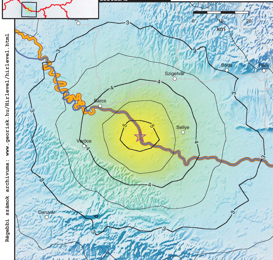
MŰSZERES ADATOKBÓL SZÁMÍTOTT INTENZITÁS ELOSZLÁS
